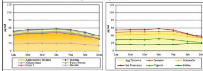
Figura 4-2: NO 2 - settimana tipica
