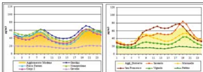
Figura 4-1: NO 2 - giorno tipico
