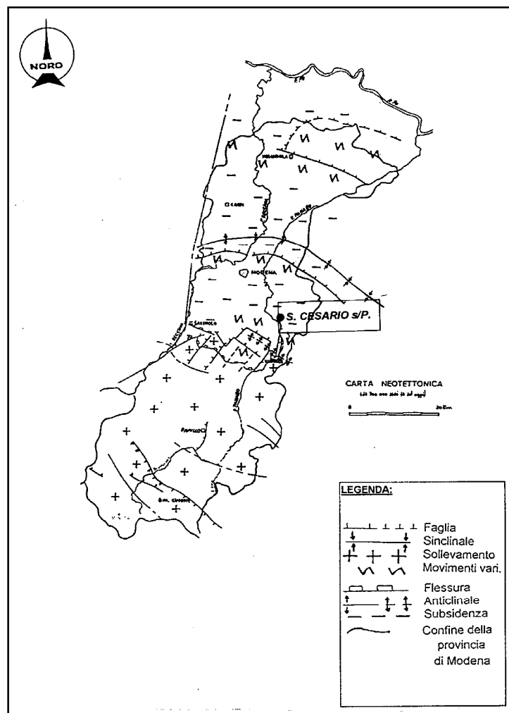
Figura 5 – Neotettonica
