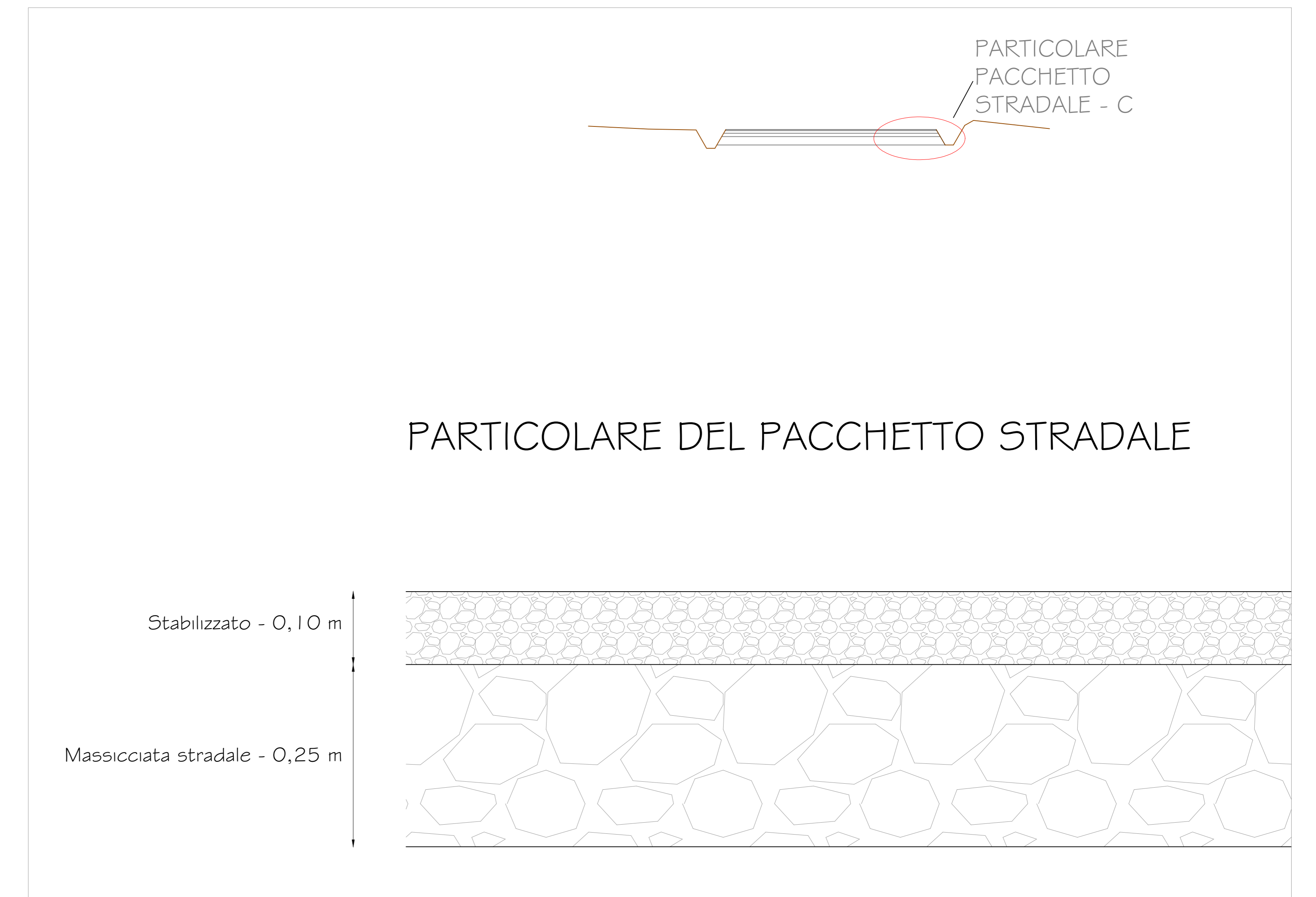
Particolare del pacchetto stradale - Scala grafica
