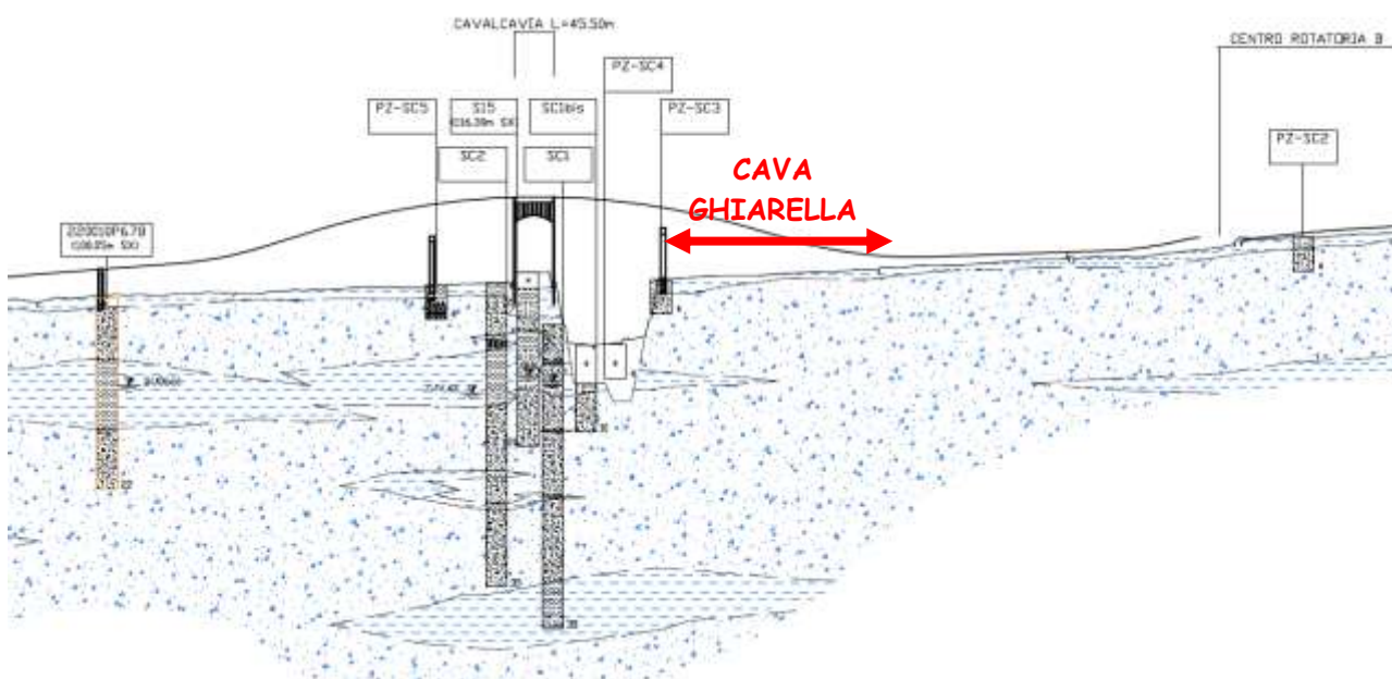
Fig. 6 - Sezione stratigrafica N-S (in asse alla futura tangenziale)
