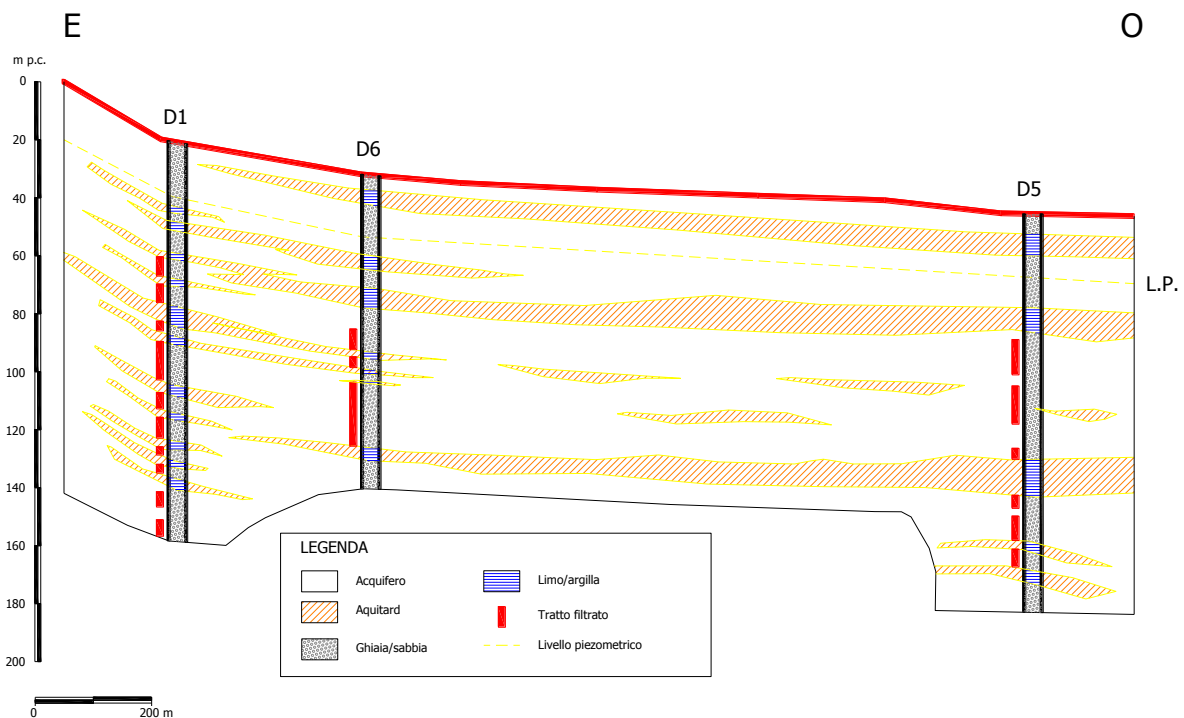
Fig. 4 - Sezione idro-stratigrafica con identificazione degli acquiferi della zona
